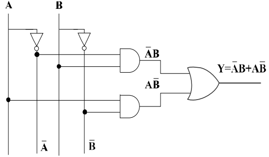
চিত্র: মৌলিক গেইট দিয়ে X-OR গেইট বাস্তবায়ন।
